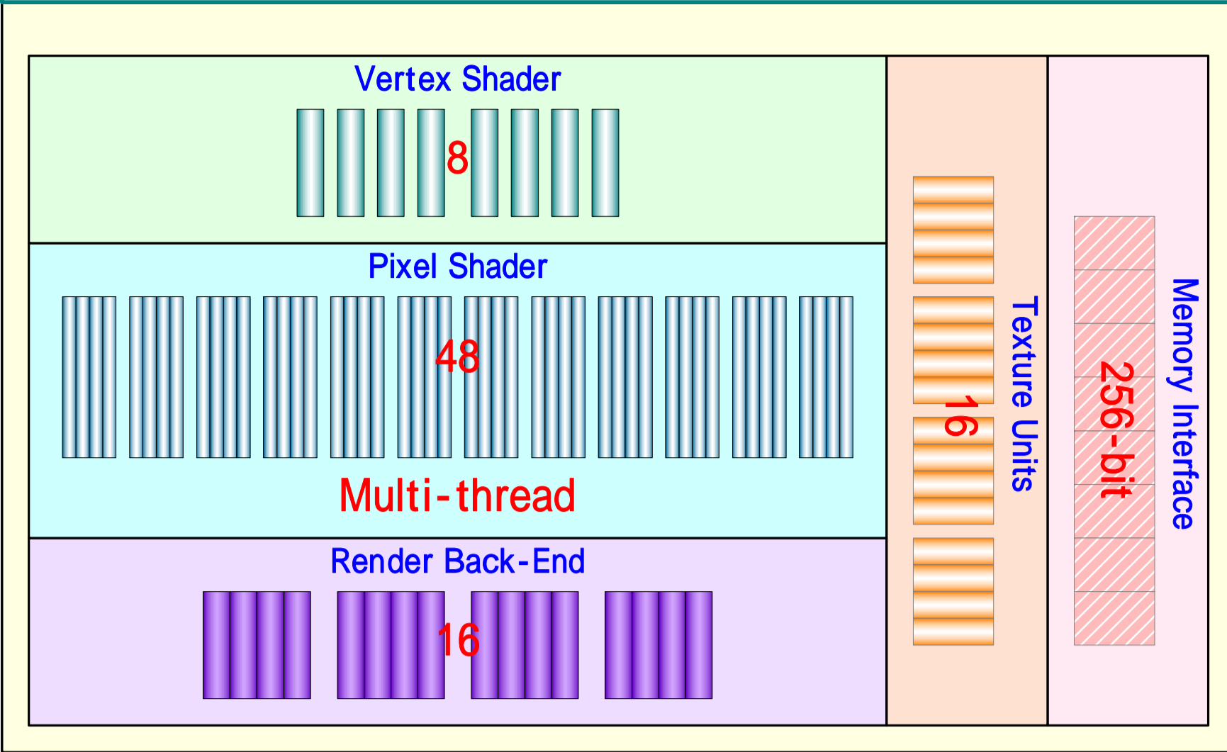
RADEON X1900 (R580)
