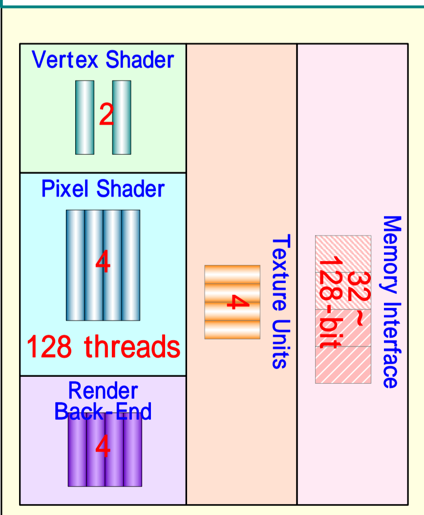
RADEON X1300 (RV515)
