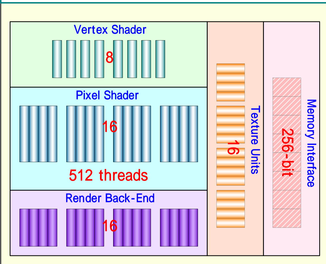
RADEON X1800 (R520)
